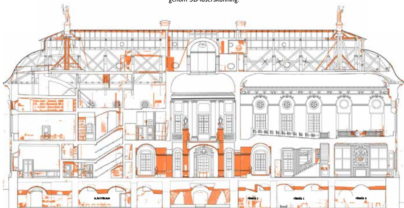
Digital sektionsritning genom riddarhuspalatset upprättad genom 3D-laserskanning.
